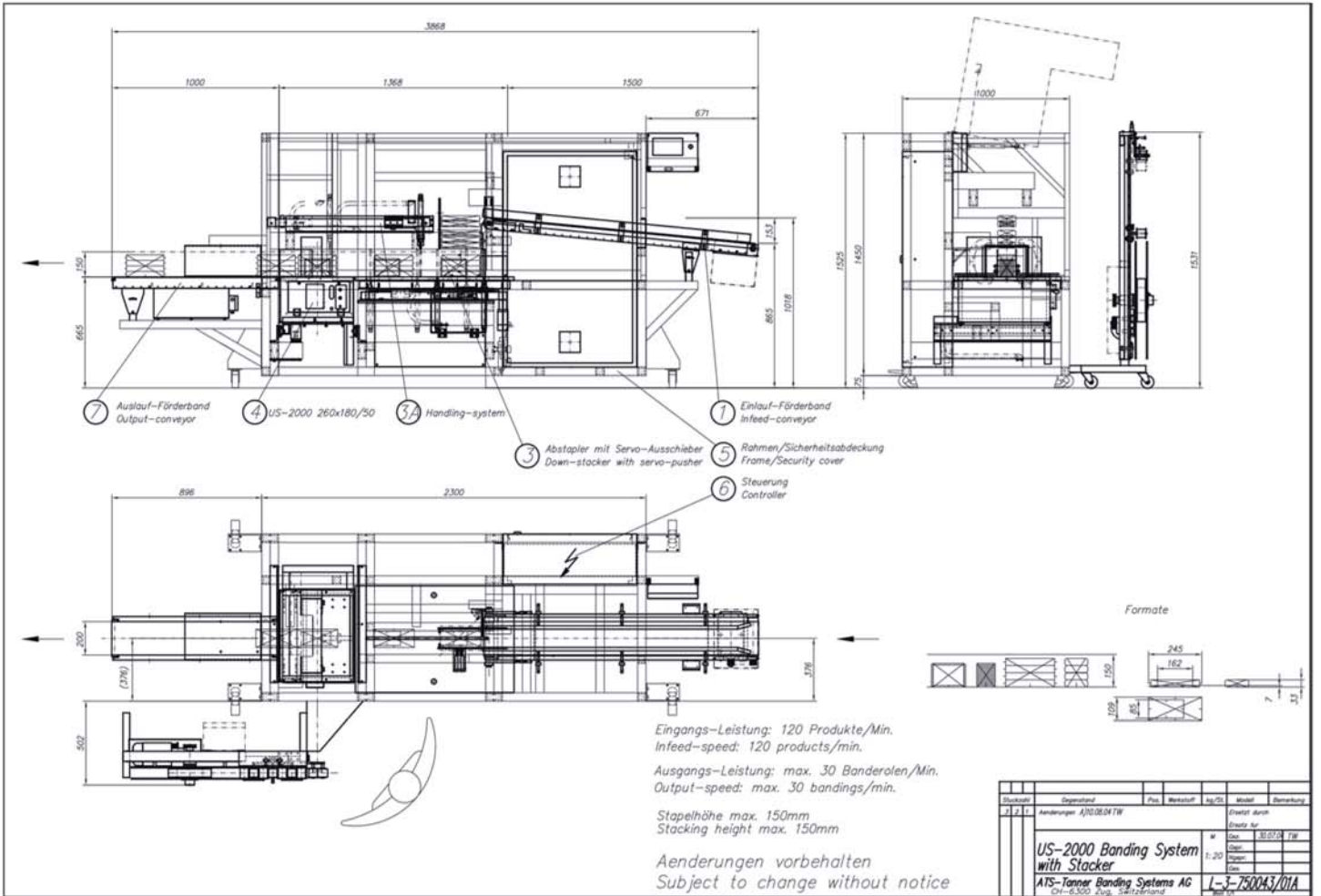
Die Produkte werden mit Zwischenstapler gestapelt. The products get stacked with intermediate stacker.
